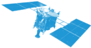
はやぶさ2
